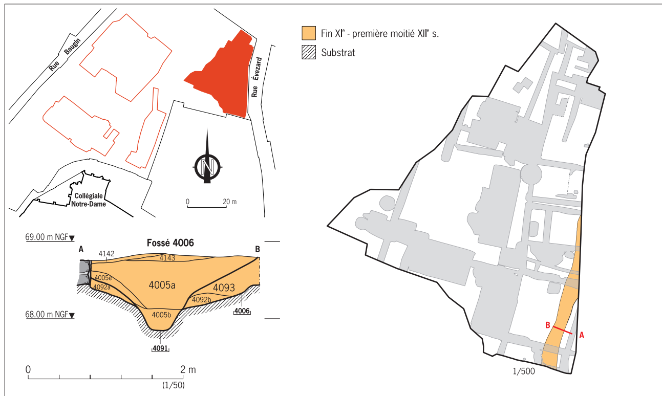
Fig. 82 Coupes du fossé bordier 4006-4091.
