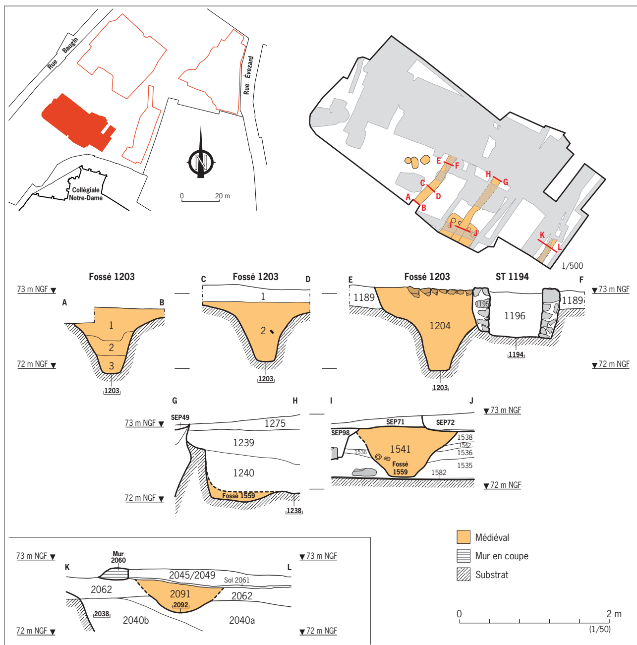
Fig.41 Coupes des fossés parcellaires.
