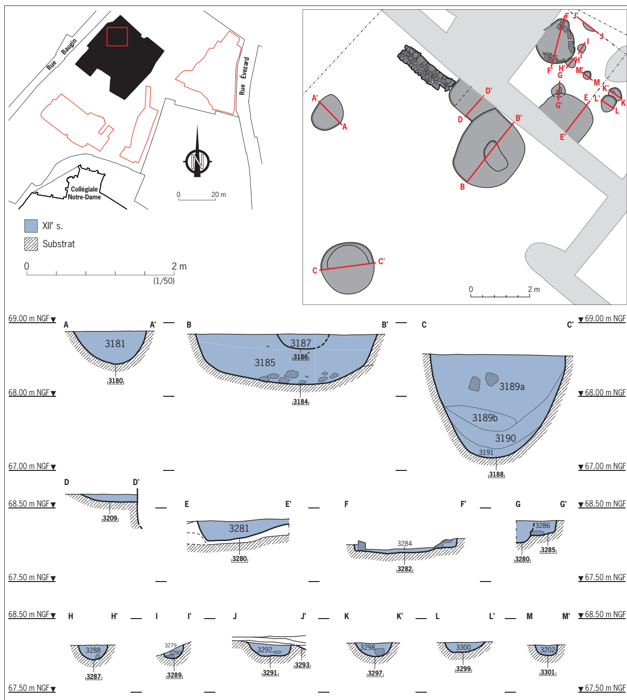
Fig. 101 Ensemble de structures en creux à l'ouest du bassin, coupes. DAO : Julia Wilson (Inrap)
