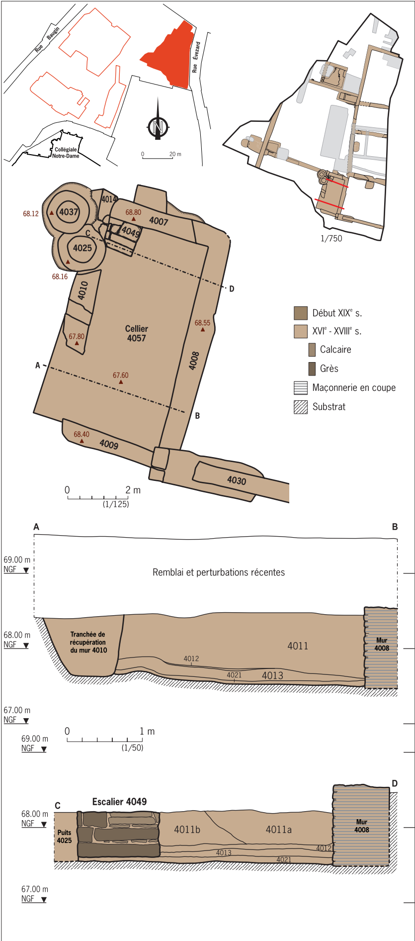
Fig. 171 Coupes stratigraphiques du cellier 4057. DAO : Steve Glisoni et Julia Wilson (Inrap)
