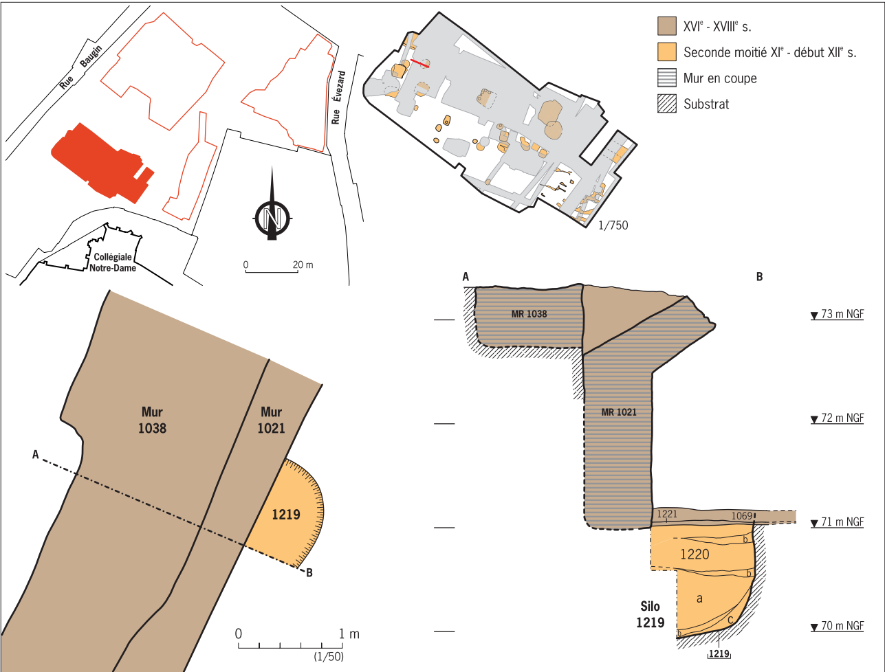
Fig. 50 Le silo 1219. DAO : Julia Wilson (Inrap)
