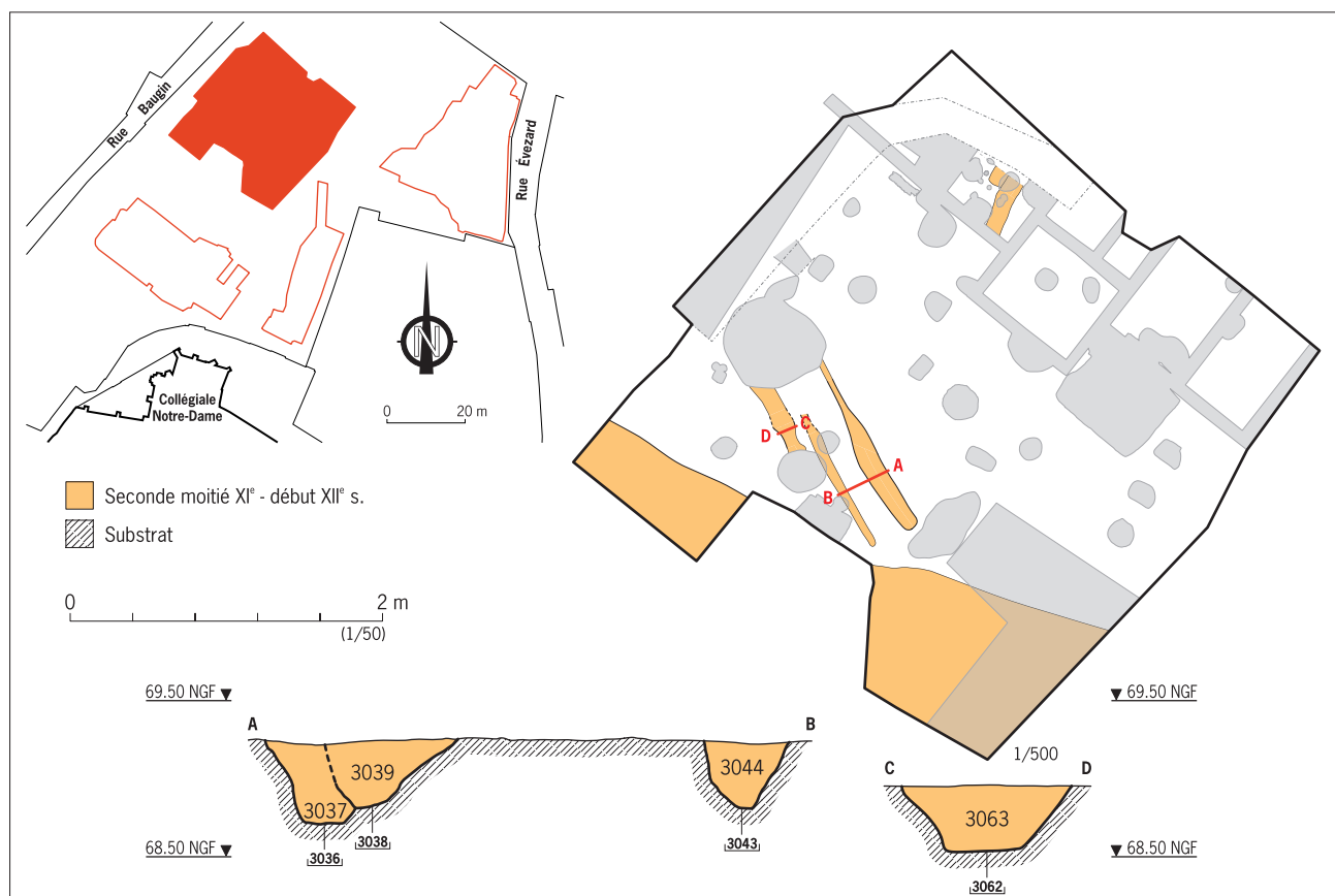
Fig. 81 Coupes des fossés parcellaires 3062-3036 et 3038-3048. DAO : Julia Wilson (Inrap)
