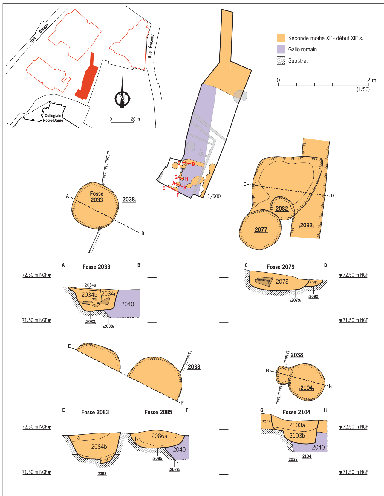
Fig.79 Fosses diverses, coupes stratigraphiques.
