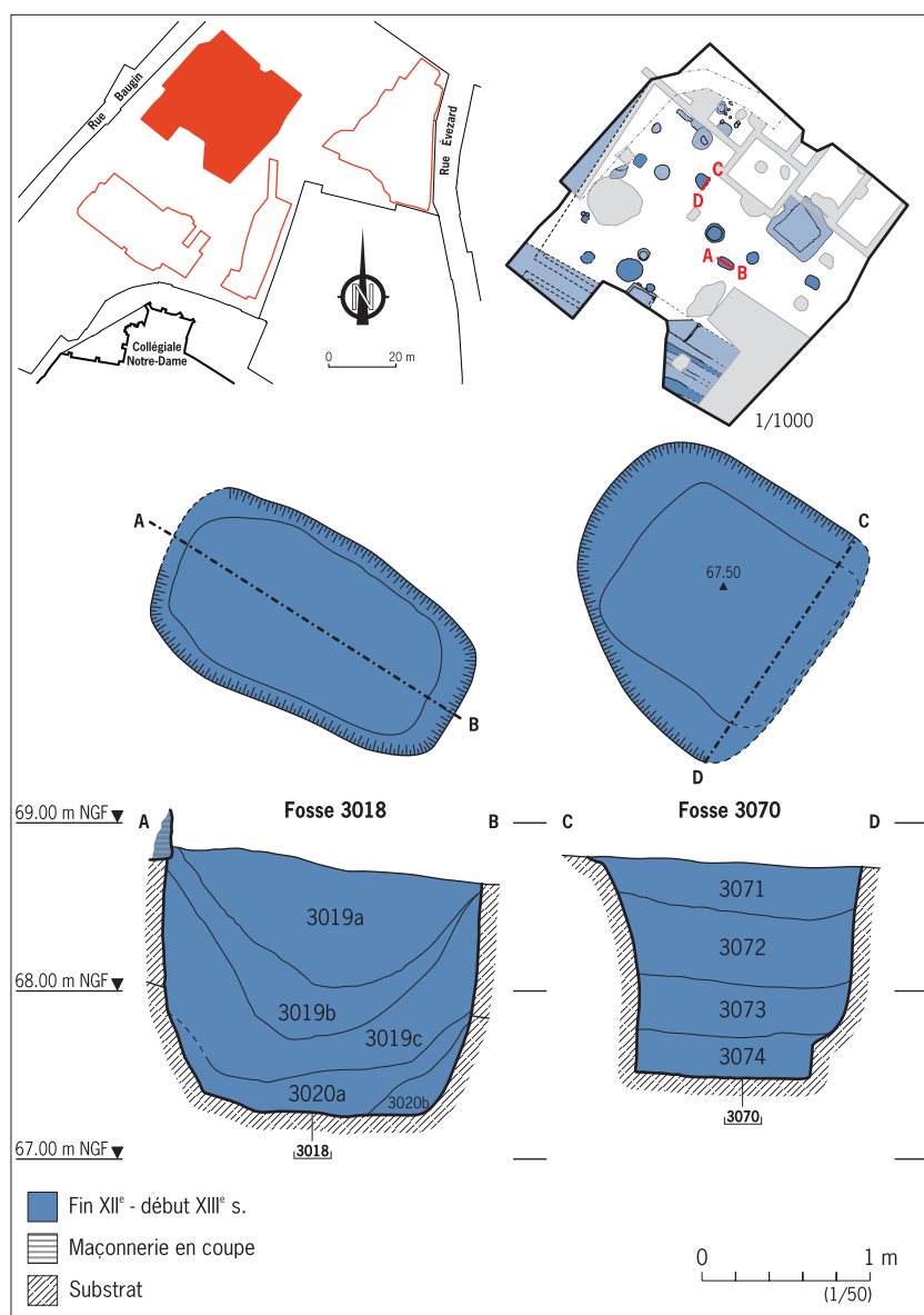
Fig. 105 Plan et coupe des fosses 3018 et 3070.
