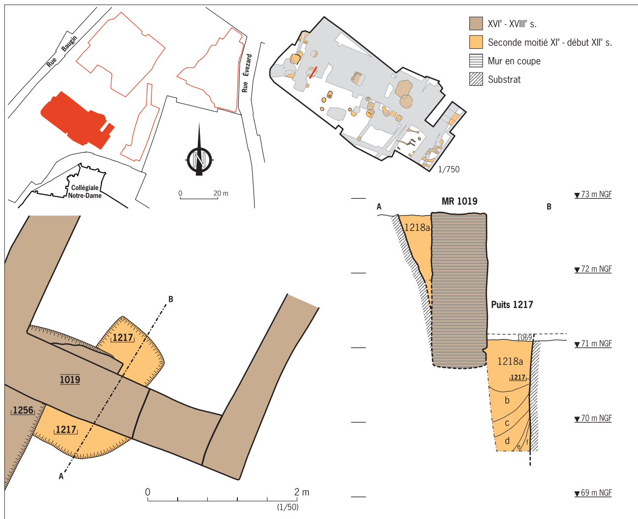
Fig. 52 Coupe du puits 1217.
